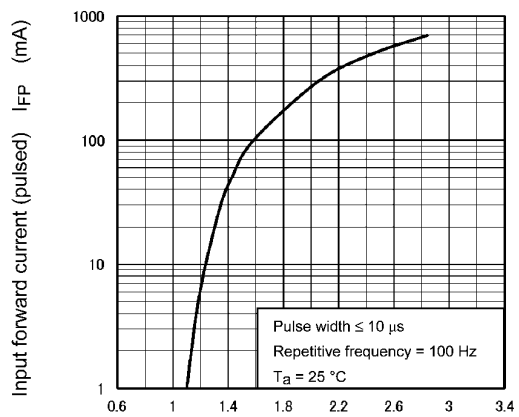
Fig. 11.6 I_{FP} - V_{FP}
