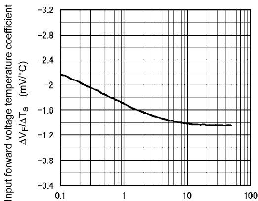
Fig. 11.5 \Delta V_F/\Delta T_a - I_F
