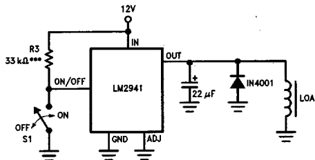
1A Switch
